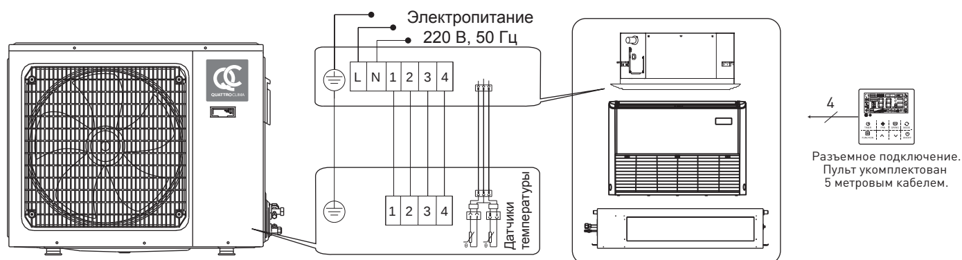
Электрическая схема QV-I18FG/QN-I18UG
