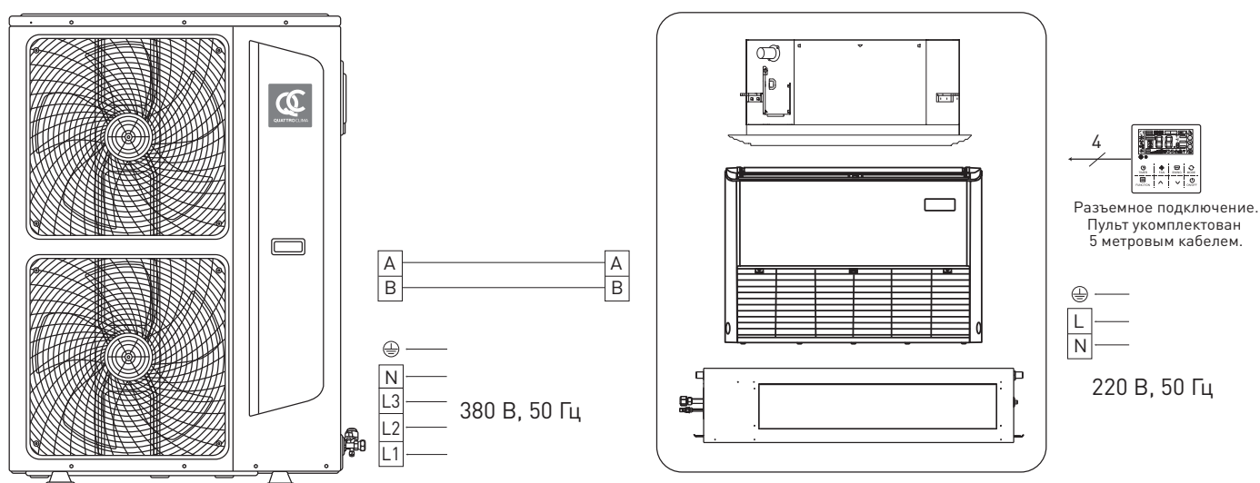
Электрическая схема QV-I36FG/QN-I36UG; QV-I48FG/QN-I48UG; QV-I60FG/QN-I60UG
