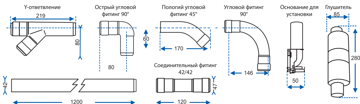
Размеры конструкции
